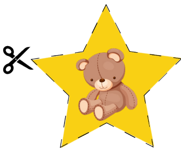
Étoiles «Objets»
